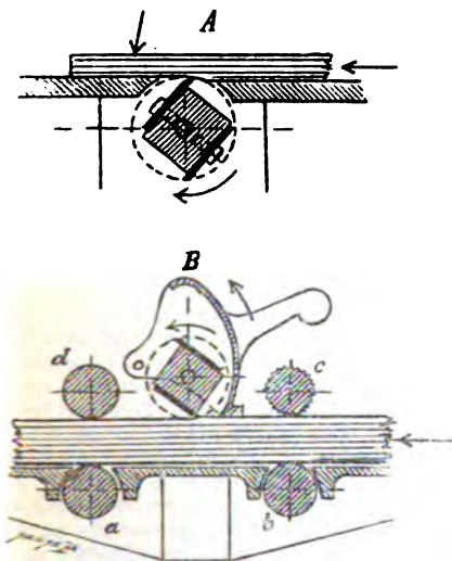
C. 1732. Hoblovací stroj na dřevo (uspořádání nožů).
